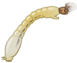
Kriebelmückenlarve
