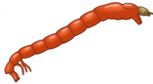
Rote Zuckmückenlarve
