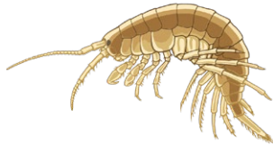
Flohkrebs
